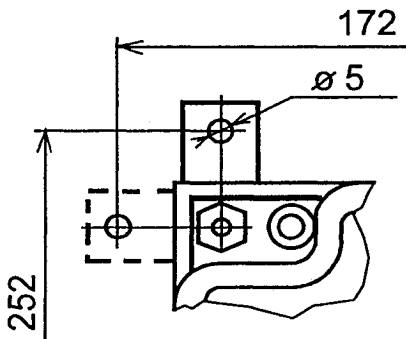
Рисунок 15 – Варианты установки кронштейнов при креплении вычислительного блока настенного исполнения.
