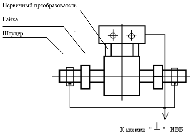
Рисунок 17 – Схема заземления первичных преобразователей.
