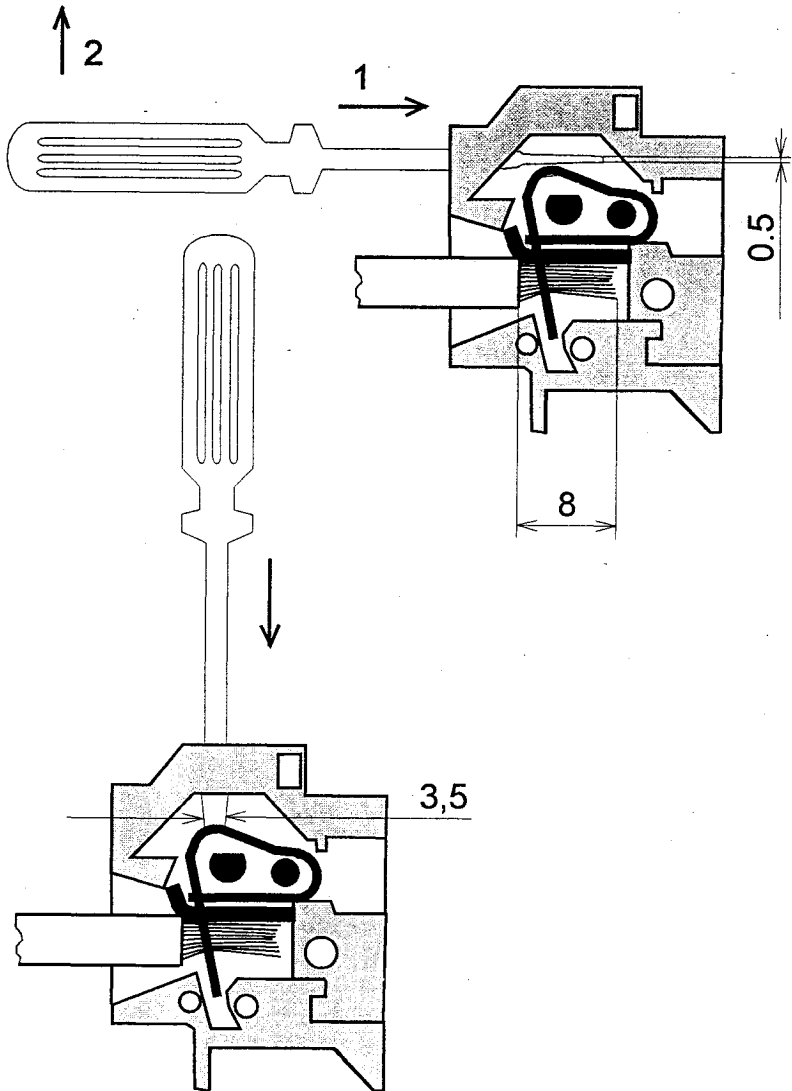
Рисунок 20 – Действия отверткой при подключении сигнальных кабелей к вычислительному блоку
