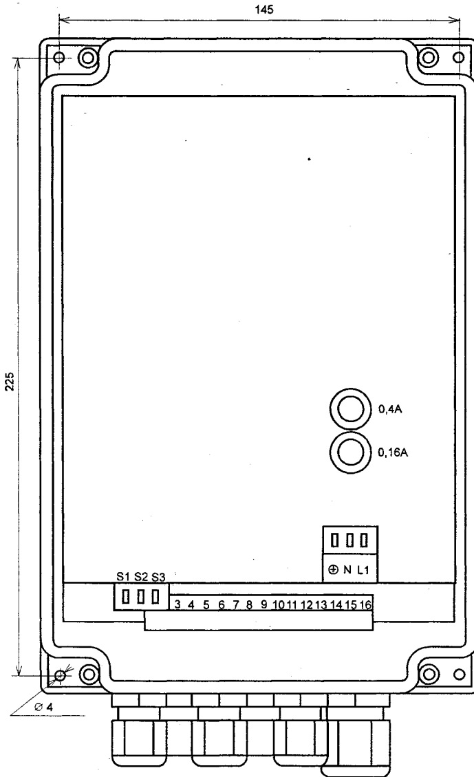
Рисунок 19 – Вид вычислительного блока настенного исполнения без крышки.
