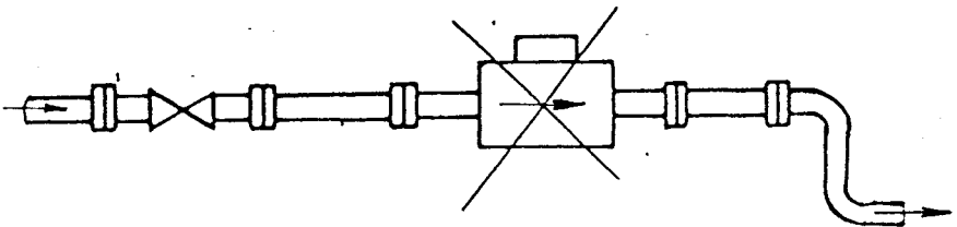
Рисунок 10 – Пример неправильной установки первичного преобразователя.
