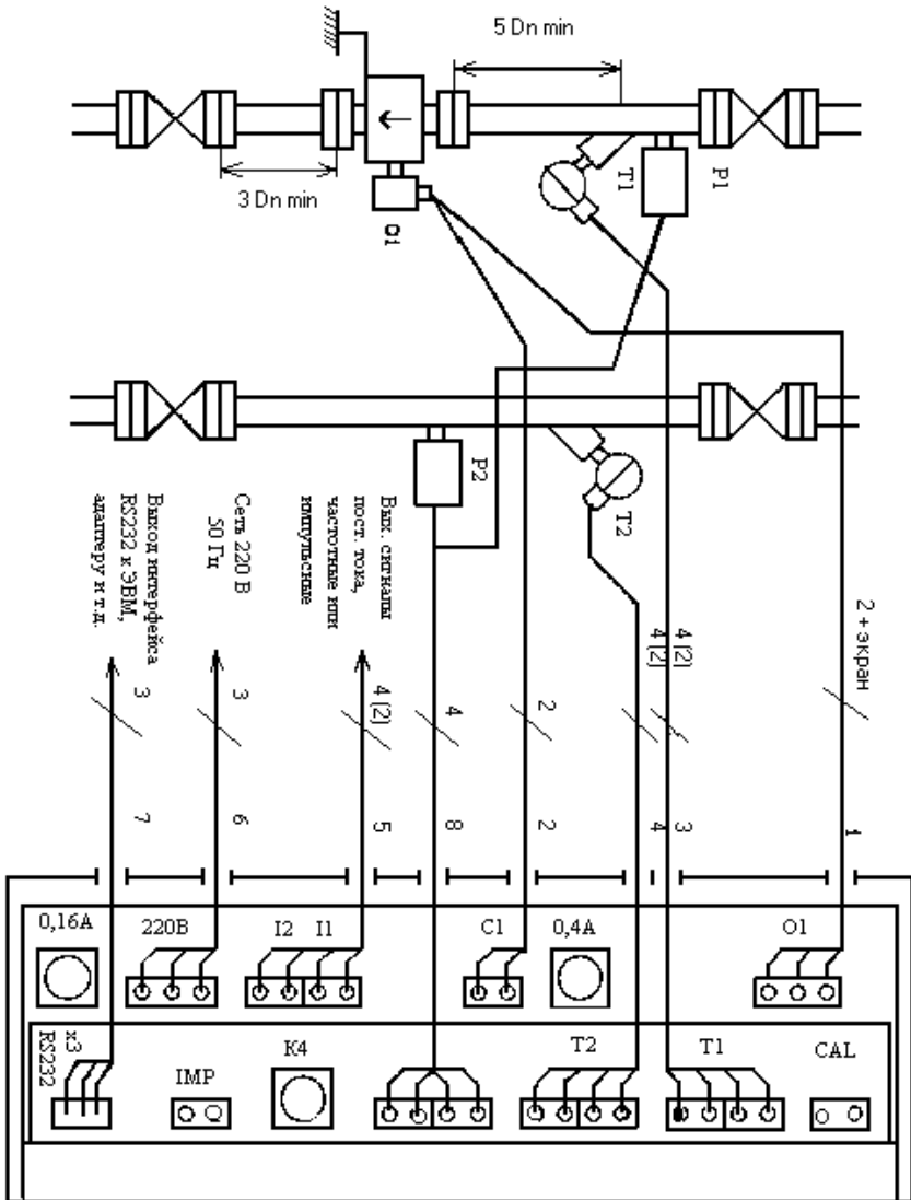
Рисунок 15 – Пример установки счетчиков ВЛР2301 на трубопроводах системы теплоснабжения
