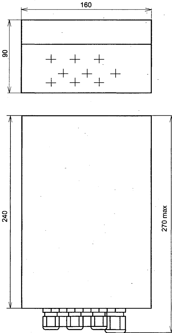
Рисунок 4 – Габаритные размеры вычислительного блока.
